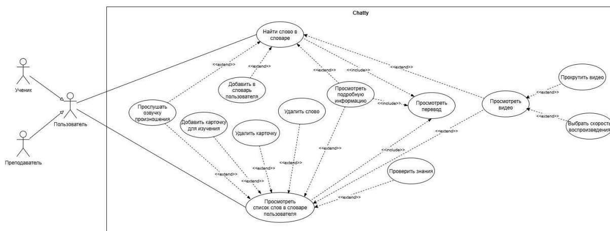
Рисунок 2. Диаграмма Use Case для версии 2.0 веб-приложения Chatty
